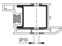
plastový profil
