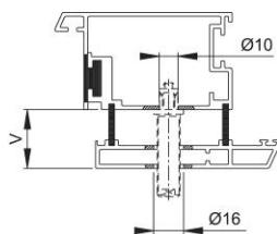
aluminium-profiel
