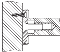
Befestigung: einseitig, mit Rosette, für Holz
