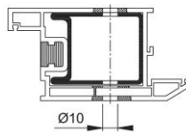
kunststof-profiel
