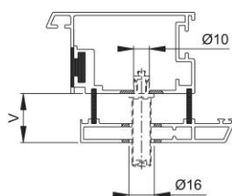
hliníkový profil
