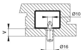
dřevěný profil
