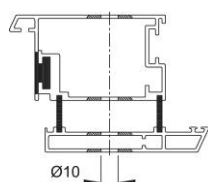
hliníkový profil
