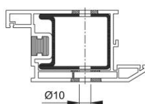
plastový profil
