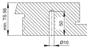
Holz-Profil
