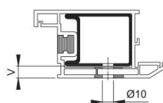
plastový profil
