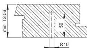
dřevěný profil
