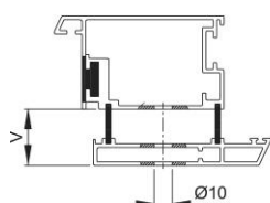
hliníkový profil
